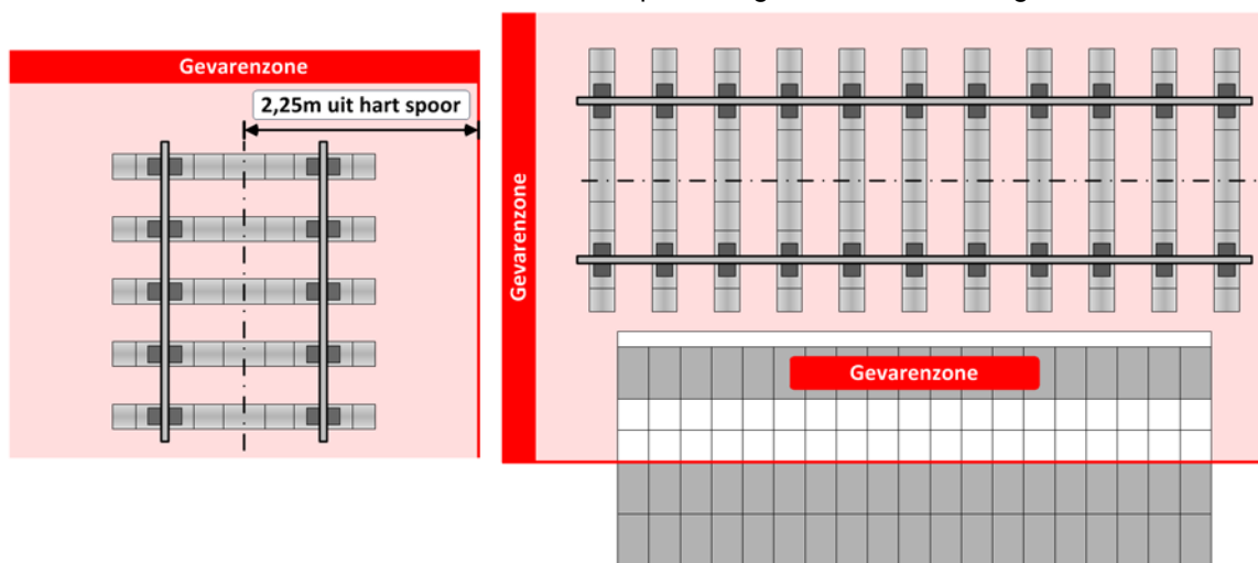
Figuur 2 - Gevarenczone Links: vrije baan en remise
